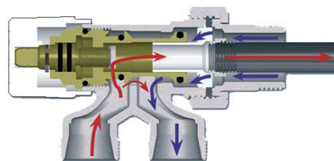
FLUSSO DI MANDATA CENTRALE
