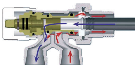
FLUSSO DI MANDATA LATERALE
